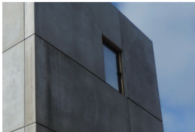
Esimerkki toleranssiluokan I seinästä.
