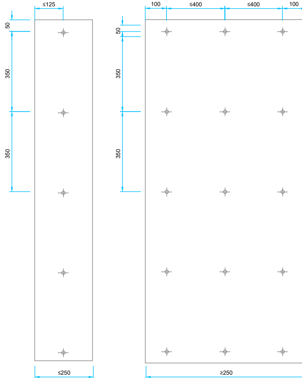
Kuva 15 (2/2). Pystysuuntainen suorakaidekanava, paloeristeenä Conlit Fire Board EI60, palonkestoluokka 60. Hitsipiikkien sijoitus
