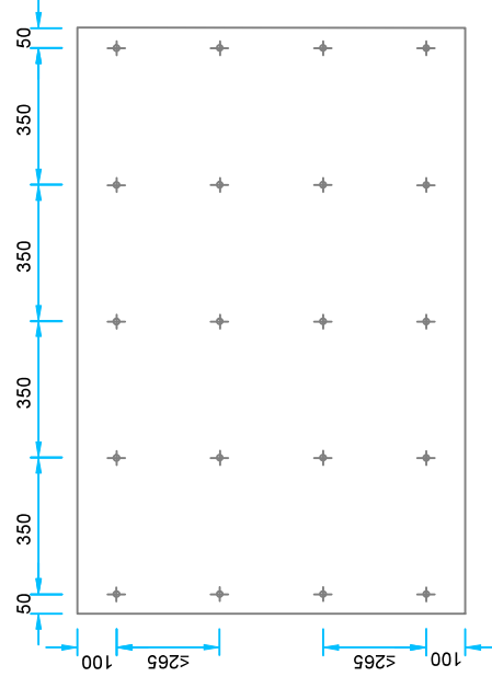
Kanavan alapuoli, hitsipiikkien maksimietäisyydet
