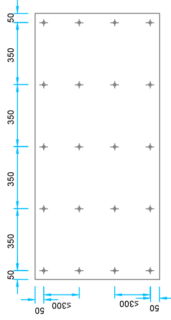
Kanavan alapuoli, hitsipiikkien maksimietäisyydet
