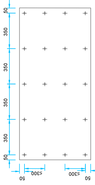
Kanavan alapuoli, hitsipiikkien maksimimäärätykset
