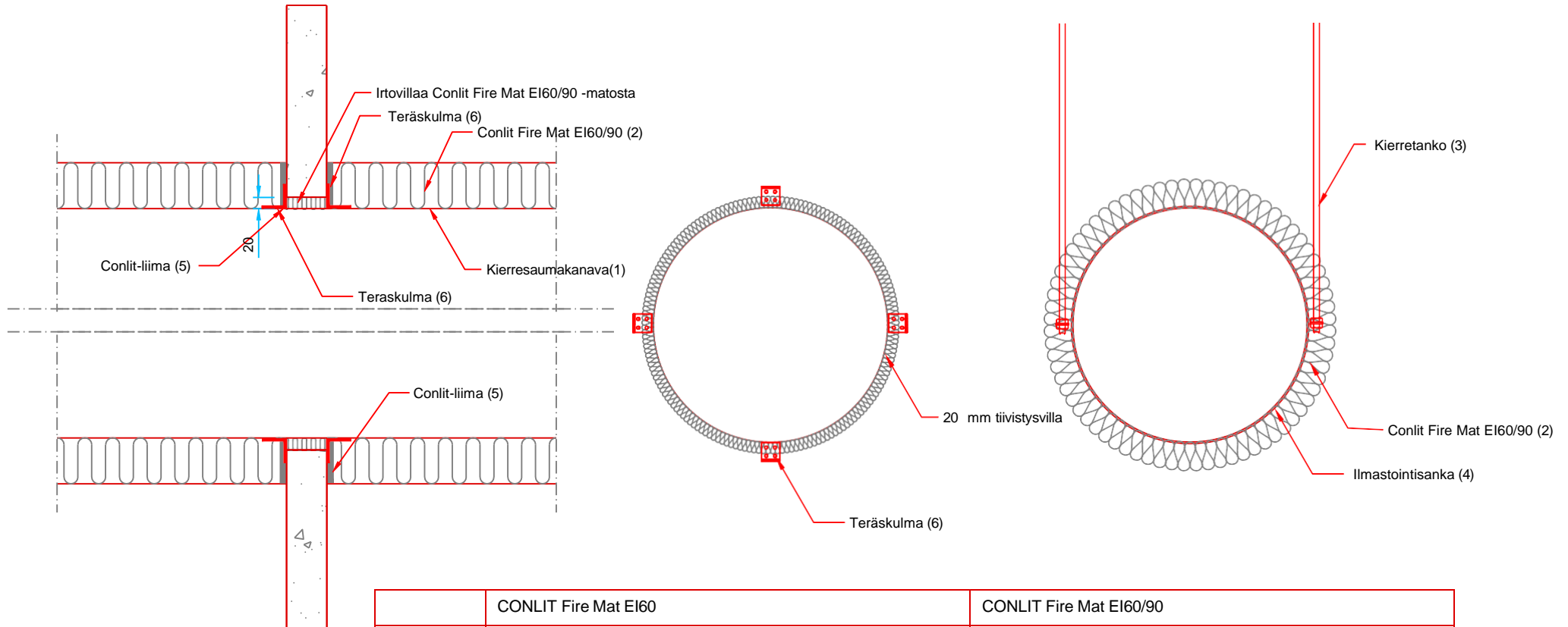
Kuva 3. Pyöreä vaakasuuntainen kanava, paloeristeenä Conlit FireMat EI60 ja Conlit FireMat EI60/90, palonkestoluokka EI 60
