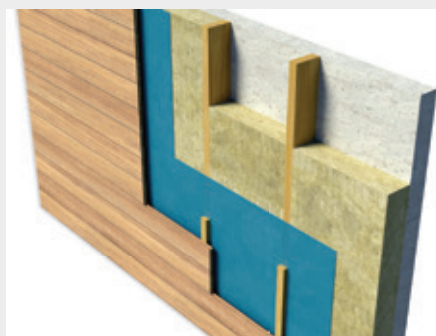
Traditioneel bevestigingssysteem met isolatie tussen houten regelwerk
