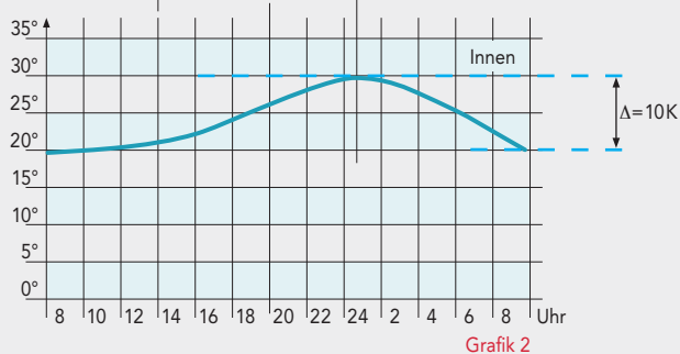
Temperaturverlauf Innenluft
