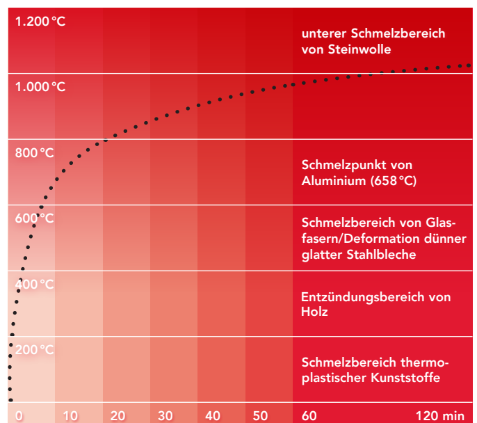
Steinwolle im Brandversuch
