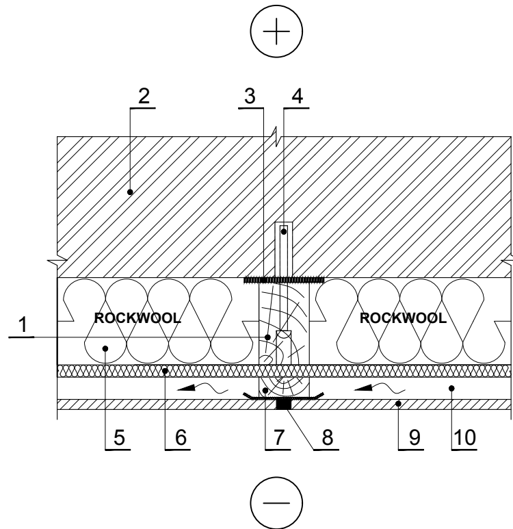
Horisontaalne sektsioon
