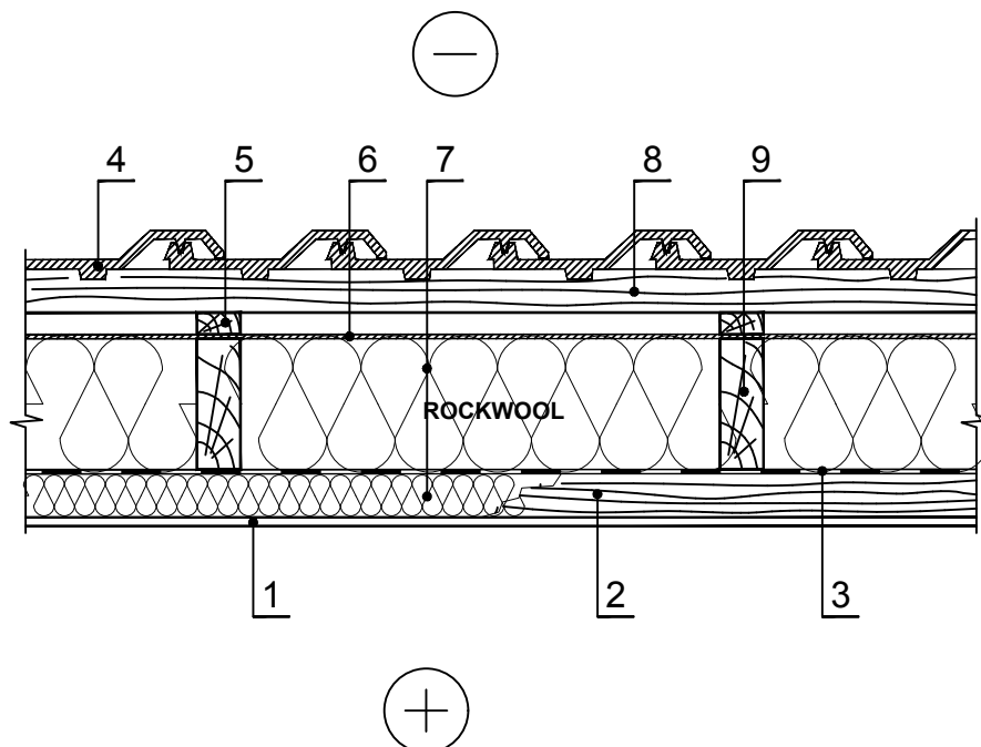
Horisontaalne sektsioon
