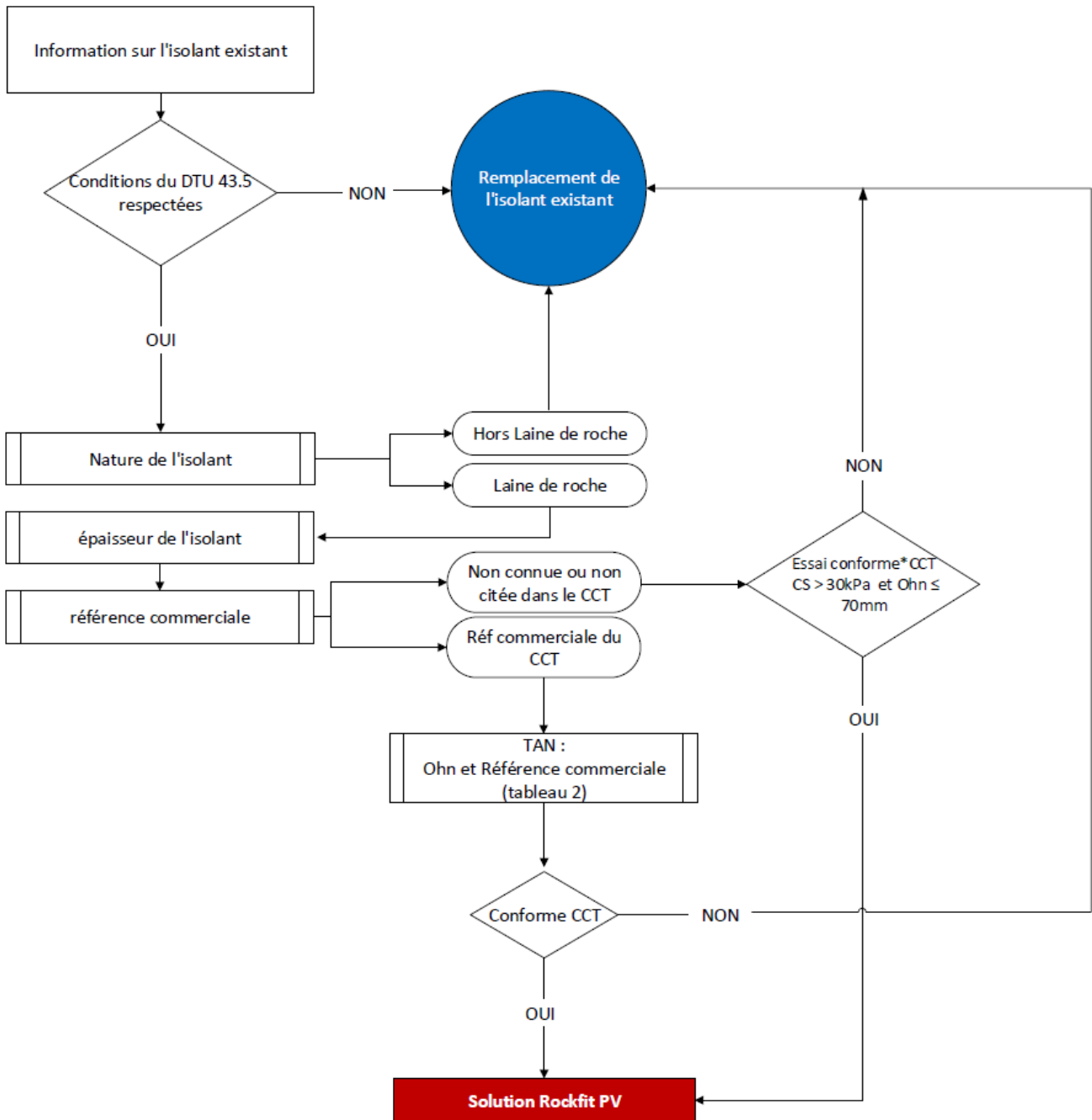
Logigramme Rockfit PV 1
