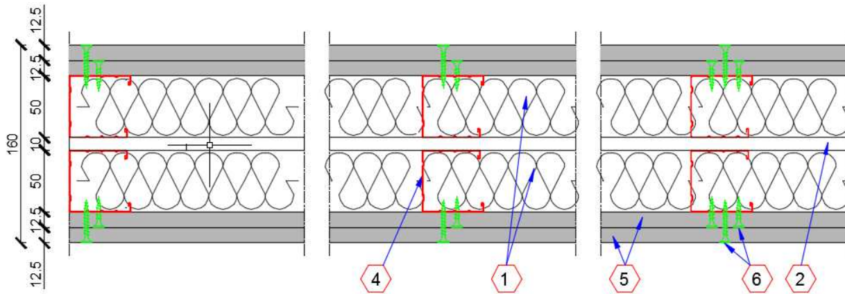
SEZIONE A - A PARTICOLARE (SCALA 1:2)
