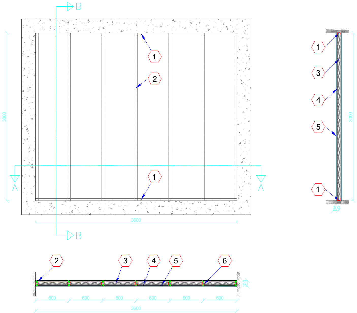
Prospetto e sezioni Elevation and sections
