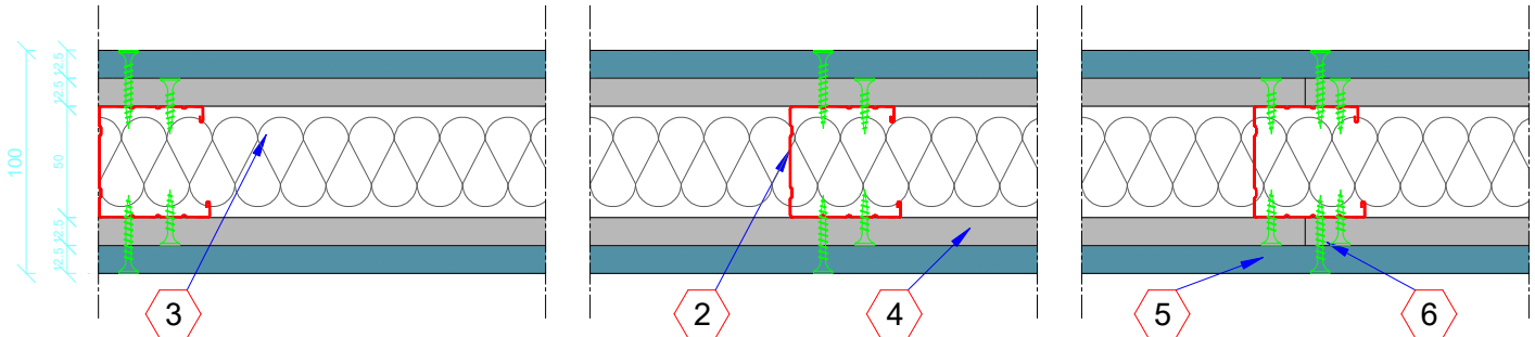
Particolare della sezione A-A Section A-A detail
