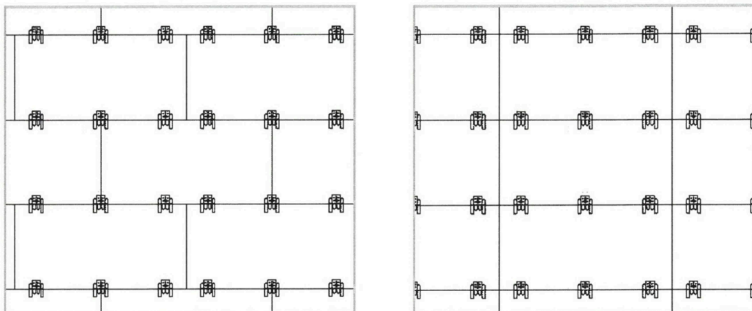
Figura 1 - Schemi di posa ganci MS 58, MS 98, MS 138 (giunti sfalsati e giunti allineati)
