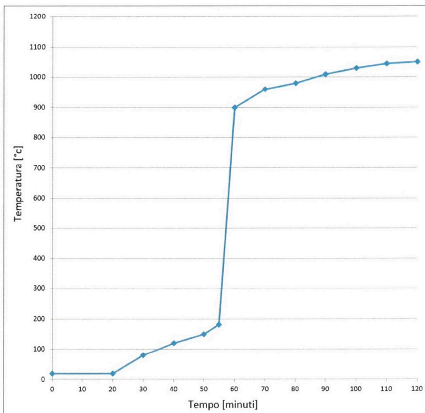
Figura 2 - curva di riscaldamento da considerarsi come condizione al contorno.
