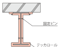
【耐風仕様】 一般部納まり例
