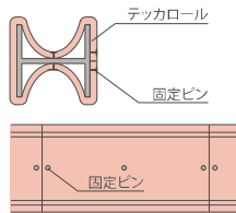
【8の字貼り仕様】
