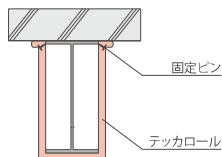
【貫通孔対応仕様】 一般部納まり例
