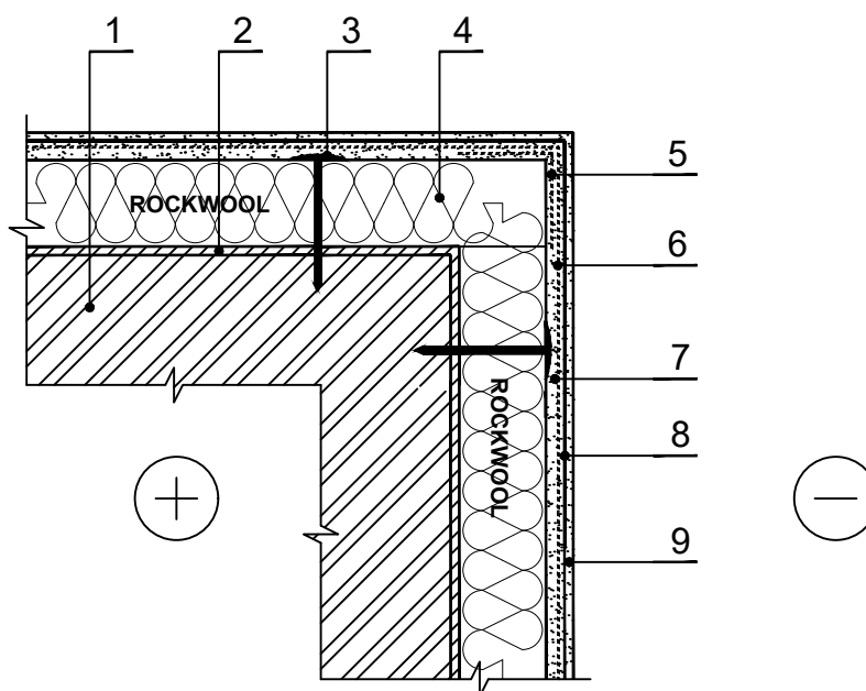
Horizontalus pjūvis
