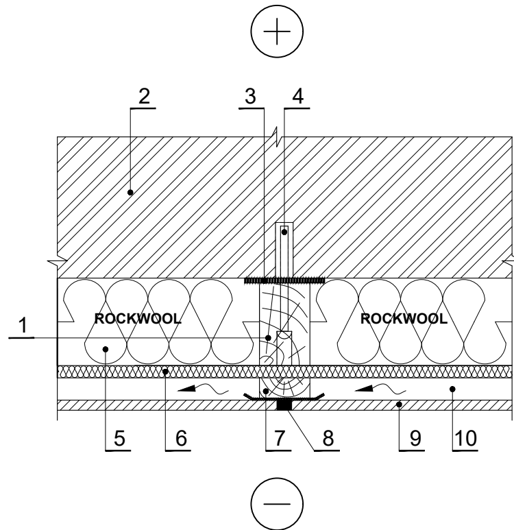
Horizontalus pjūvis
