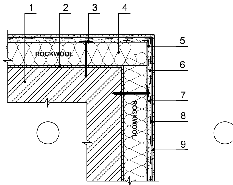
Horizontālā sadaļa
