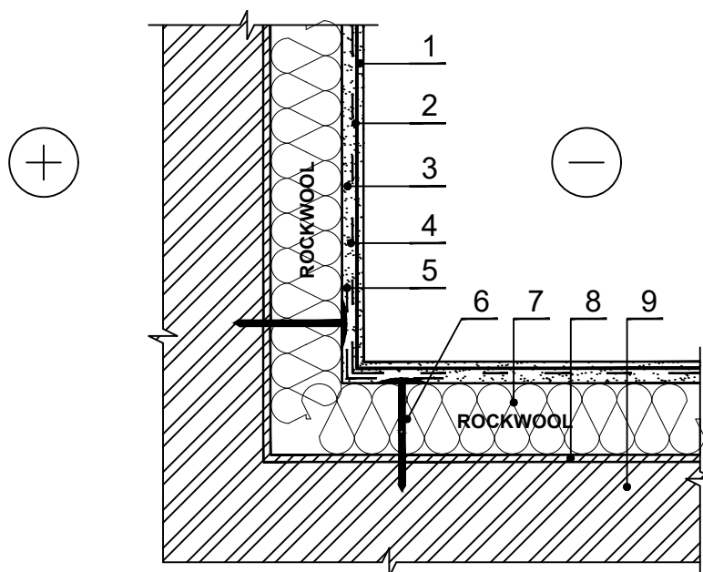
Horizontālā sadaļa
