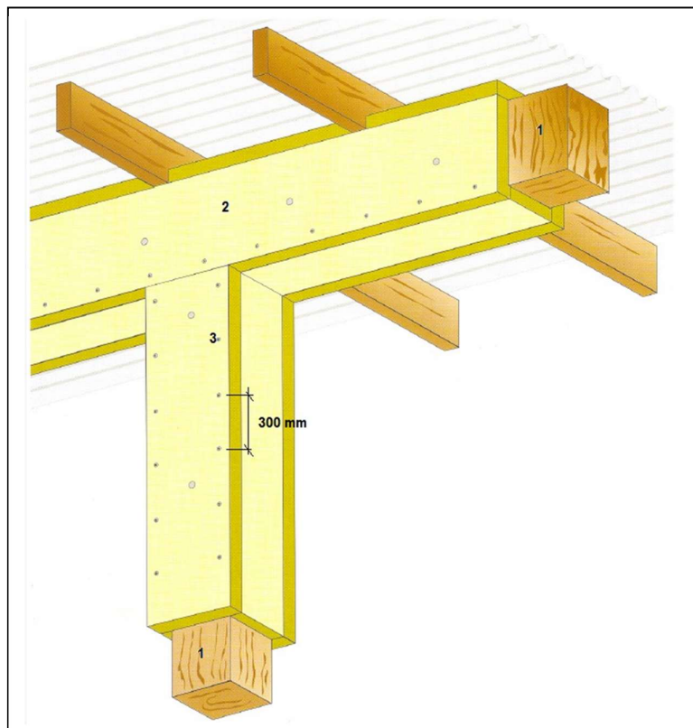
1 – koka konstrukcija; 2 – plāksnes CONLIT 150; 3 – metāla stiprinājuma elements
