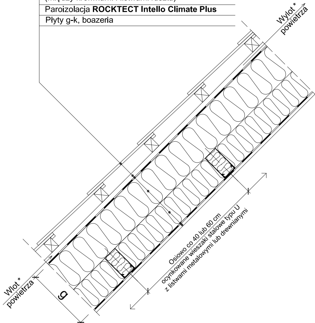
Energooszczędne ocieplenie dwuwarstwowe
