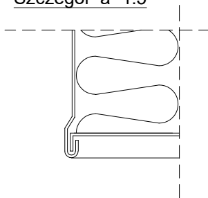
Szczegół "a" 1:5
