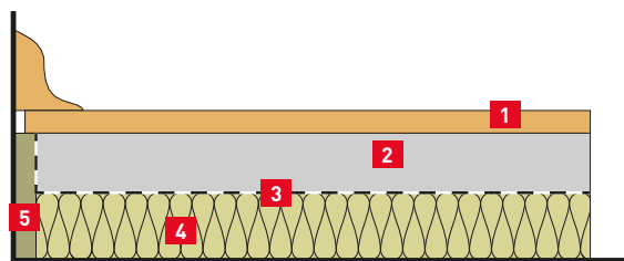
RYSUNEK 1. Izolacja podłogi pływającej na podkładzie anhydrytowym lub podkładzie cementowym
