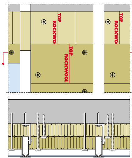
Ruszt mocowany do ściany za pomocą elementów dystansujących. Płyty wchodzą w ruszt.
